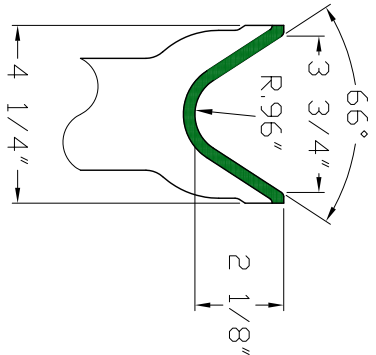
GROOVE CONFIG. (1.5 : 1)
