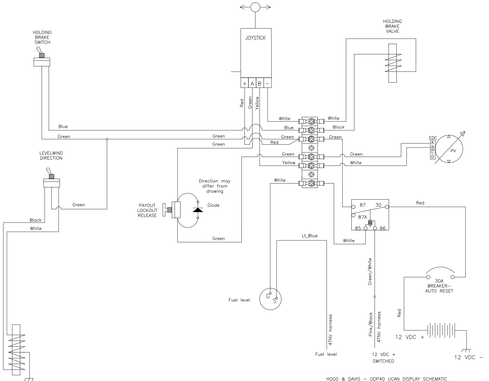
HOGG & DAVIS - ODP40 UCAN DISPLAY SCHEMATIC
