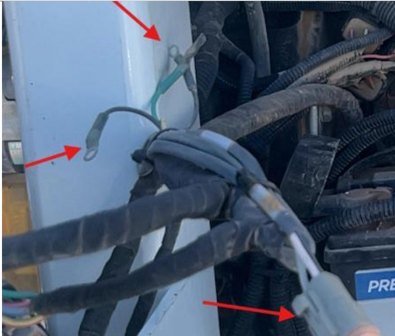
Loose Wiring
